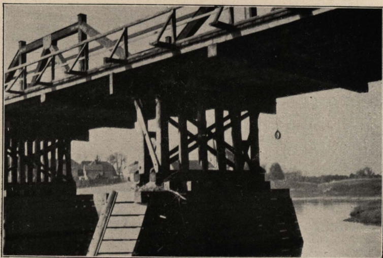
159. Pfeilerkonstruktion der neuen Warthe-Straßenbrücke in Obersitz, Kr. Samter BB 6971/Objekt 30. Dauerbehelfsbrücke aus Holz (s. Erläuterung zu Bild 158).
