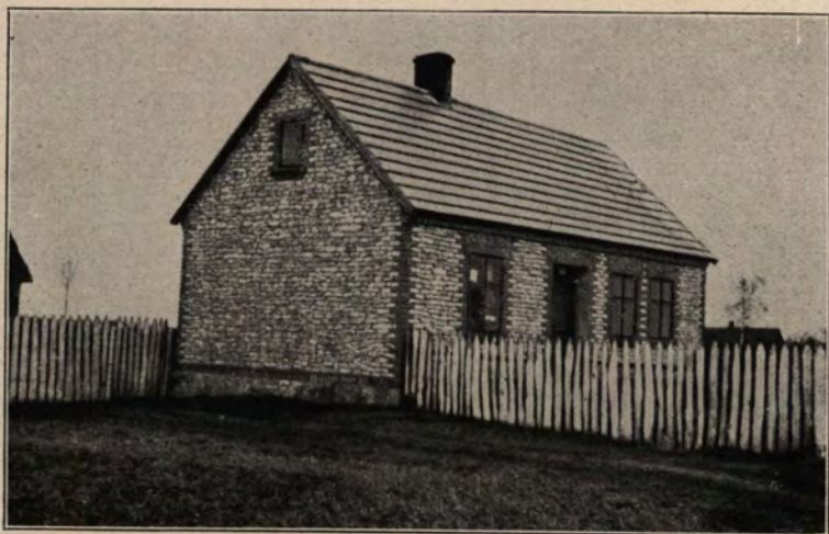
107. Haus aus Kalkstein n. Hohenbühl (Dobra), Kr. Tureck BB 7368. Auf dem Kalkuntergrund im S. O. des Warthelandes neuerdings öfter angewandte Bauweise (s. Bilder 97 und 121).
